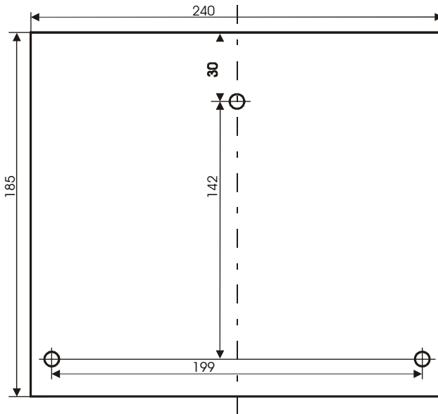
Rys. 1. Wymiary gabarytowe obudowy i rozmieszczenie otworów mocujących.
